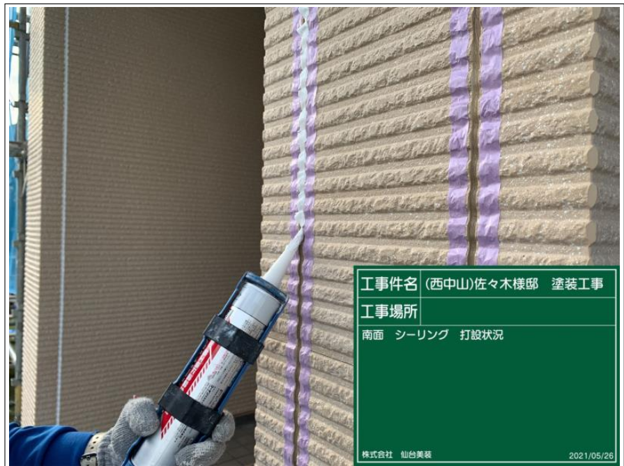
西中山 佐々木様邸 塗装工事 シーリング作業
