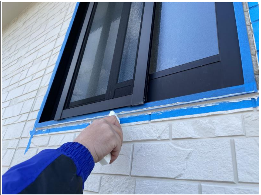
シーリング増し打ち工法
