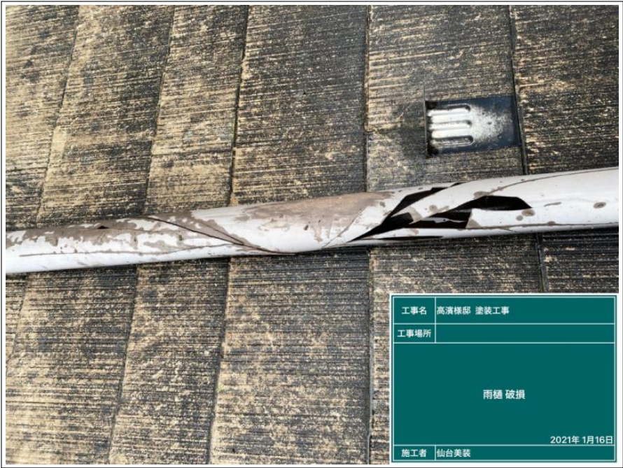
樋破損部
